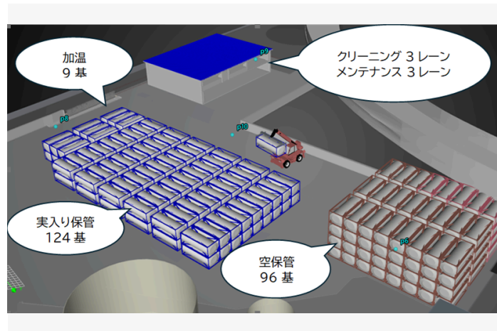
構内配置図（完成イメージ）
